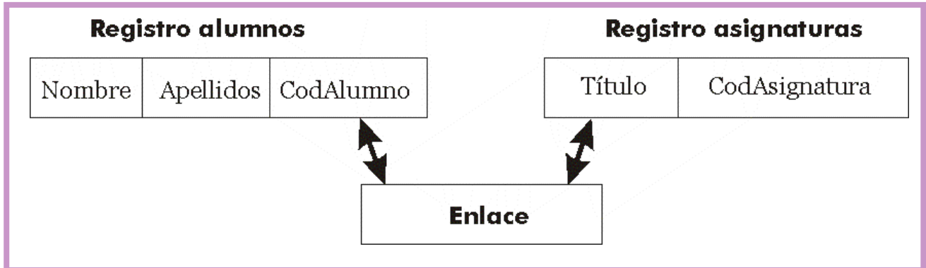
Ilustración 11, ejemplo de diagrama de estructura de datos Codasyl
